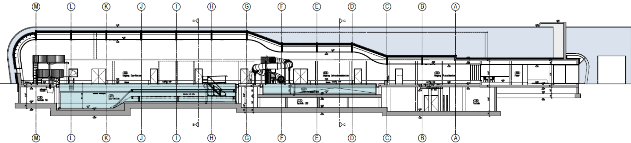
SCHNITT A-A
