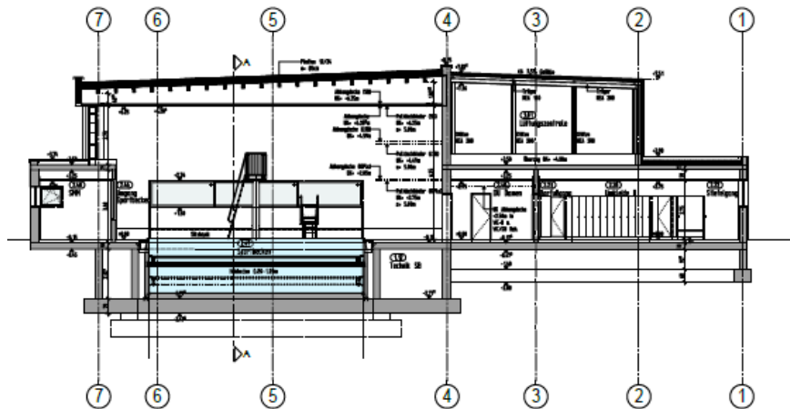
SCHNITT B-B
